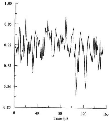
图 2 500 hPa 信号场通过正态性显著检验 (5% 显著水平) 网格点所占比例随日数变化
