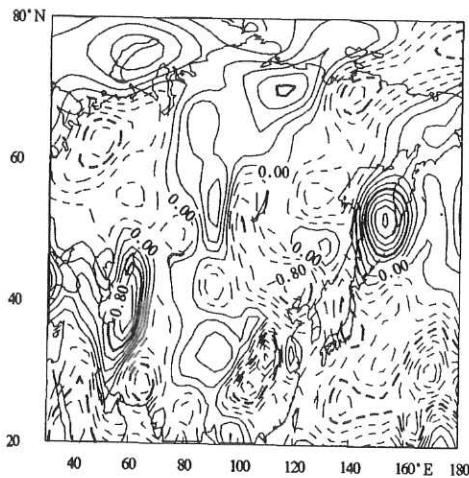
图 1 5 月 11 日 500 hPa 信号场各格点的偏度系数分布
