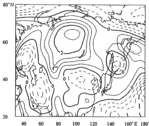
图3 1992年5月15日原500 hPa信号场
