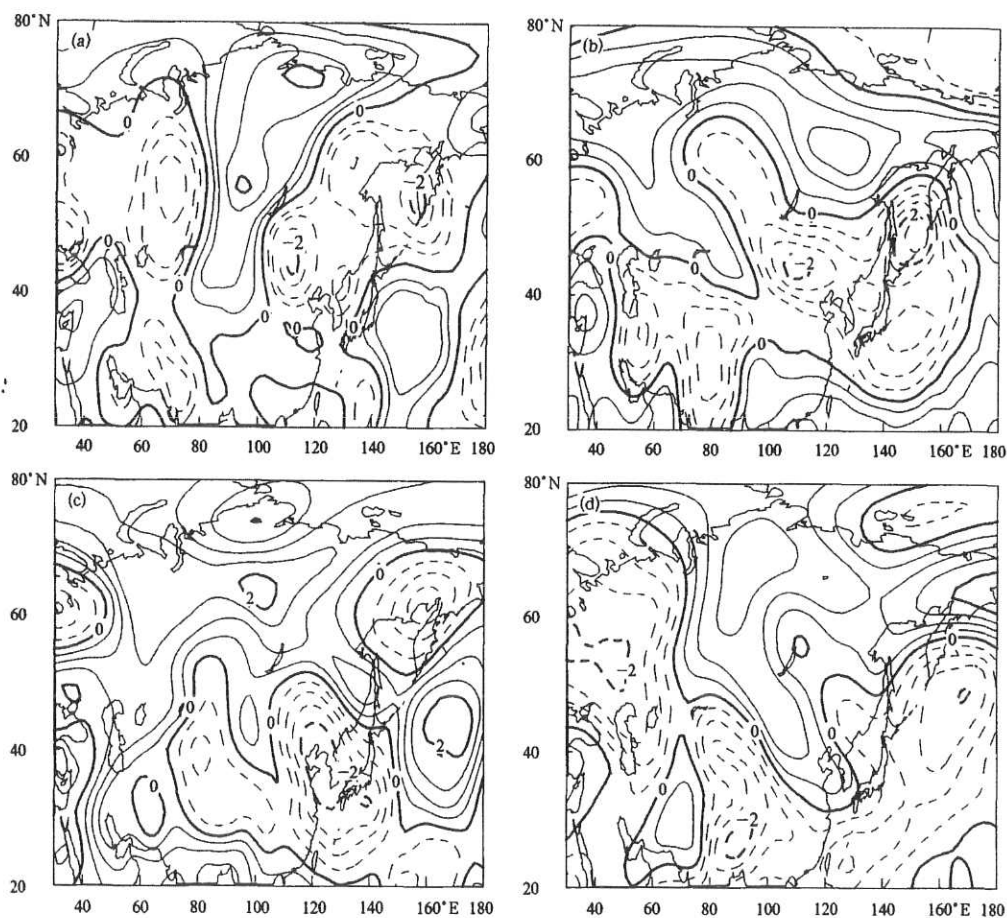
图 7 暴雨过程第 1 天的 500 hPa 信号场比较
