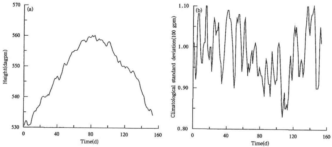
图 6 70°N 纬圈平均气候背景场汛期逐日变化过程曲线 (a. 气候平均场逐日变化, b. 气候标准差( \sigma )场逐日变化)
