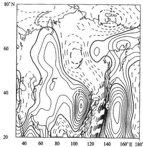
图 9 无雨日 500 hPa 信号场合成 r 值 Fig. 9 The field of r -values during the days of no rain
