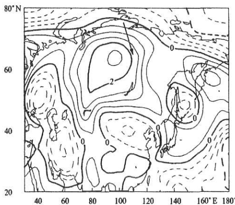
图4 1992年5月15日变换后的500 hPa信号场
